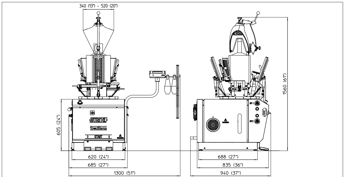
Figura 2.2 – Medidas de la máquina (en mm y pulgadas)
